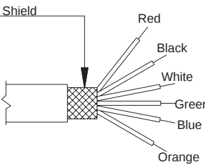
F - 6 pole cable
