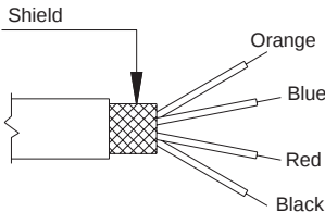
F - 4 pole cable
